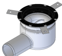
Ablaufkörper horizontal mit Geruchverschluss
