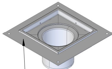
Aufsatzstück mit Klebeflansch 50mm, mit sekundär- entwässerung 413127
