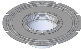
Verlängerung mit Klebeflansch 408216
