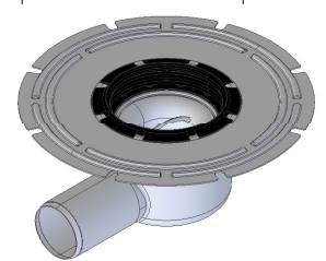
Ablaufkörper horizontal mit GV und Klebeflansch
